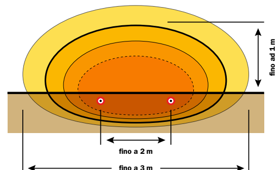
Dimensioni del campo di rilevamento MicroTrack™ II
